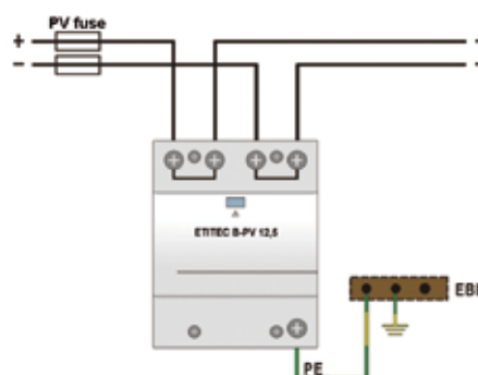
Conexión V ETITEC B-PV V connection ETITEC B-PV
