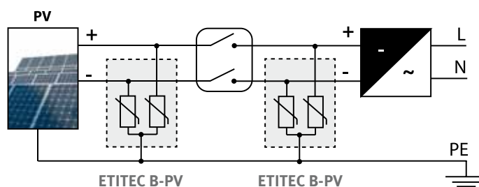
ETITEC B-PV 1000/ 12,5 (10/350)
