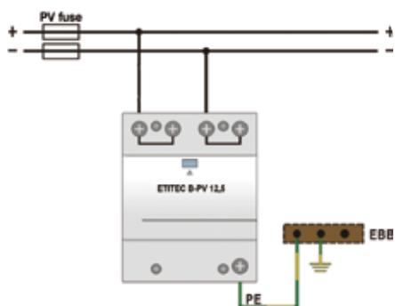
Conexión T ETITEC B-PV T connection ETITEC B-PV
